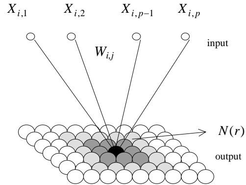
Fig. 2 SOM Neural Network
